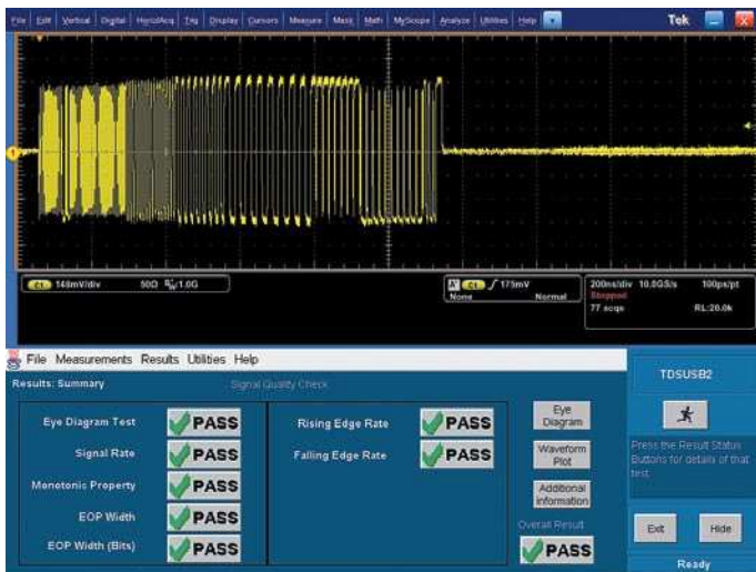
Тестирование на соответствие USB 2.0.
