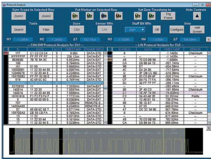
Временные соотношения и декодировка протоколов CAN и LIN.
